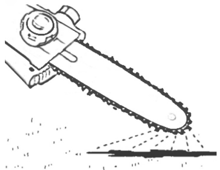
Fig. 9 – Comprobar el funcionamiento del sistema de lubricación
