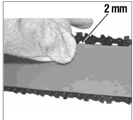
Fig. 7 – Verificando o ajuste da corrente
