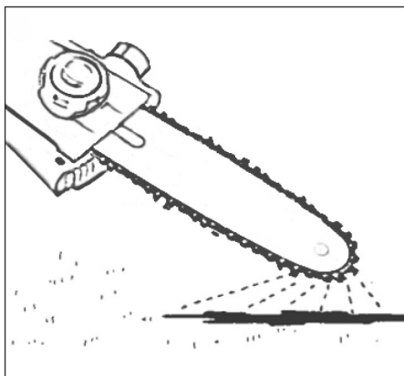
Fig. 10 – Verificar o funcionamento do sistema de lubrificação
