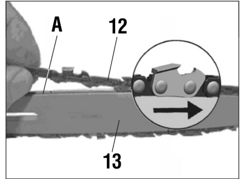
Fig. 3 – Instalación de la cadena
