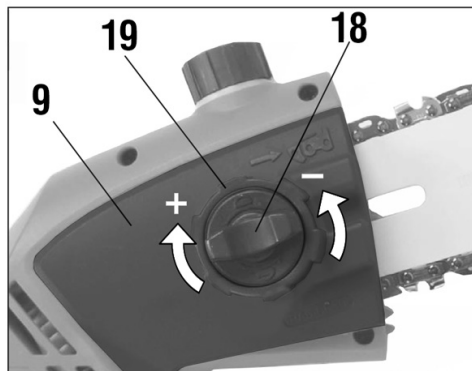
Fig. 6 – Pino tensor de la cadena
