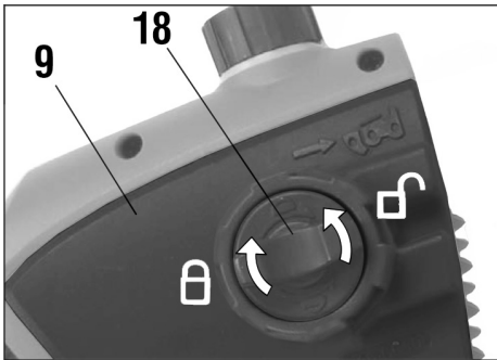
Fig. 2 – Abrir y cerrar la tapa de protección del sable
