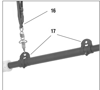
Fig. 13 – Sistema de fijación del cinturón
