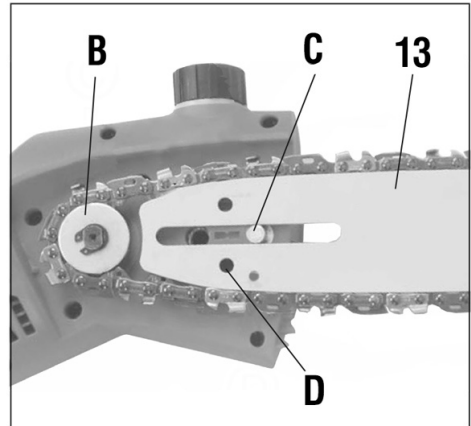
Fig. 4 – Posicionando la cadena y el sable
